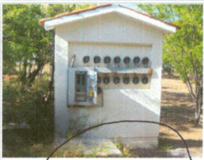
F3: Área para instalación de Wathorímetros
