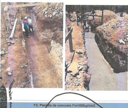
F3: Plancha de concreto f'c=100kg/cm2
