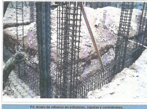
F4: Acero de refuerzo en columnas, zapatas y contratabres.
