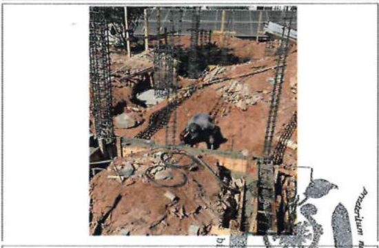
COLOCACIÓN Y CUBRADO DE CIMENTOS, ZAPATAS CORRIDAS Y AISLADAS
